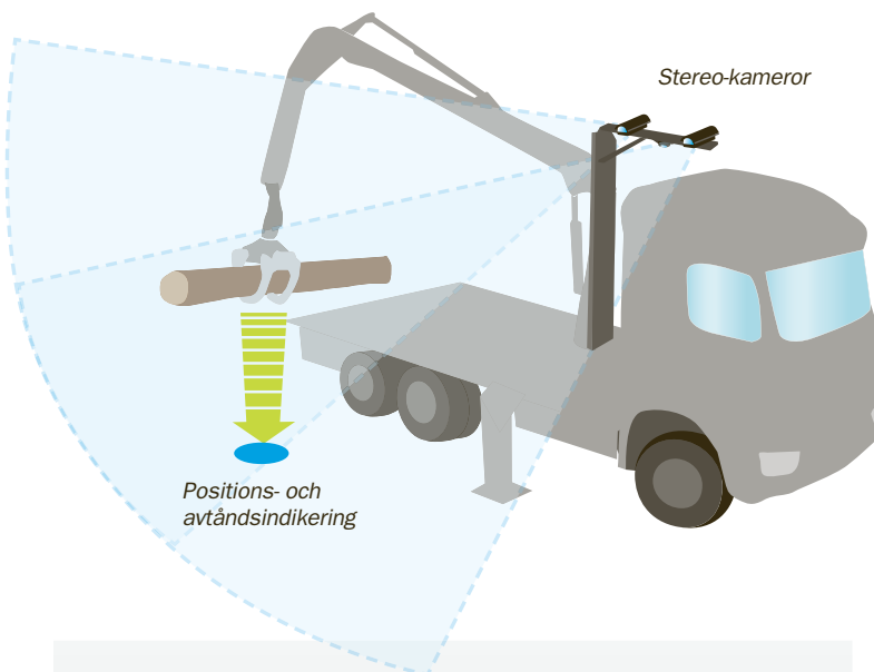
Skärmbild: En blå punkt som indikerar gripens exakta vertikala placering, samt avståndet till stockarna, syns alltid på skärmen.
