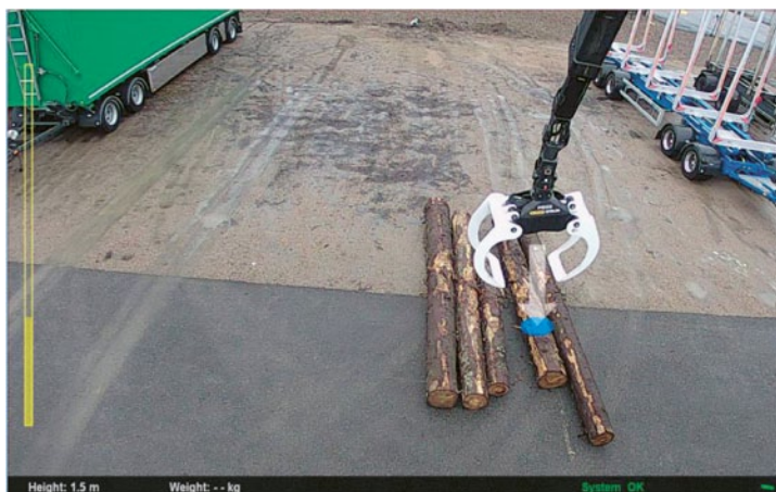
Skärmbild: En blå punkt som indikerar gripens exakta vertikala placering, samt avståndet till stockarna, syns alltid på skärmen.
